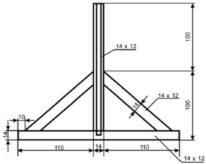
Secțiune A-A
